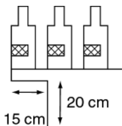
Figuur 2. Minimale voertruimte voor een stelling.
